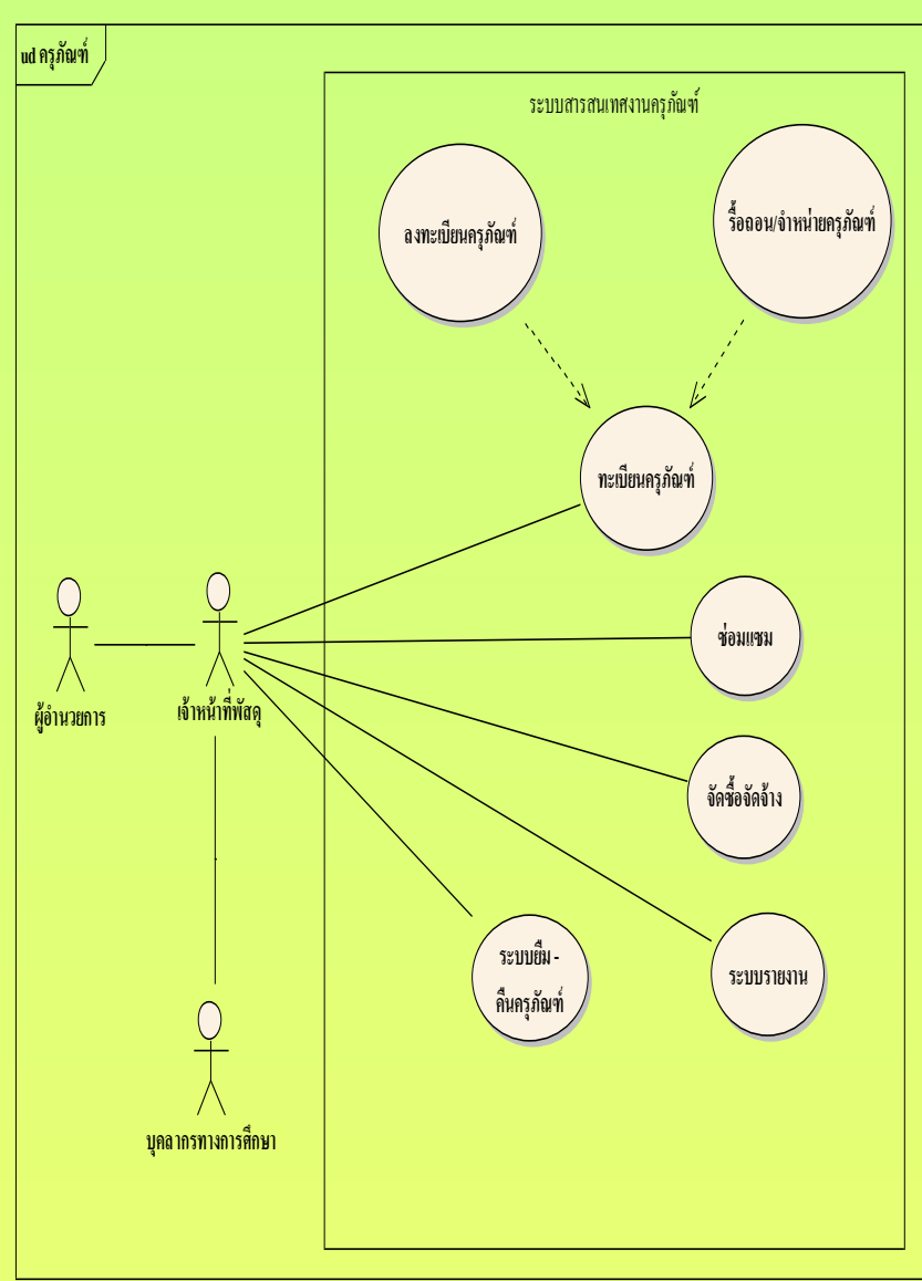
Use Case Diagram ของระบบสารสนเทศงานครุภัณฑ์โรงเรียนบ้านสองคอน
